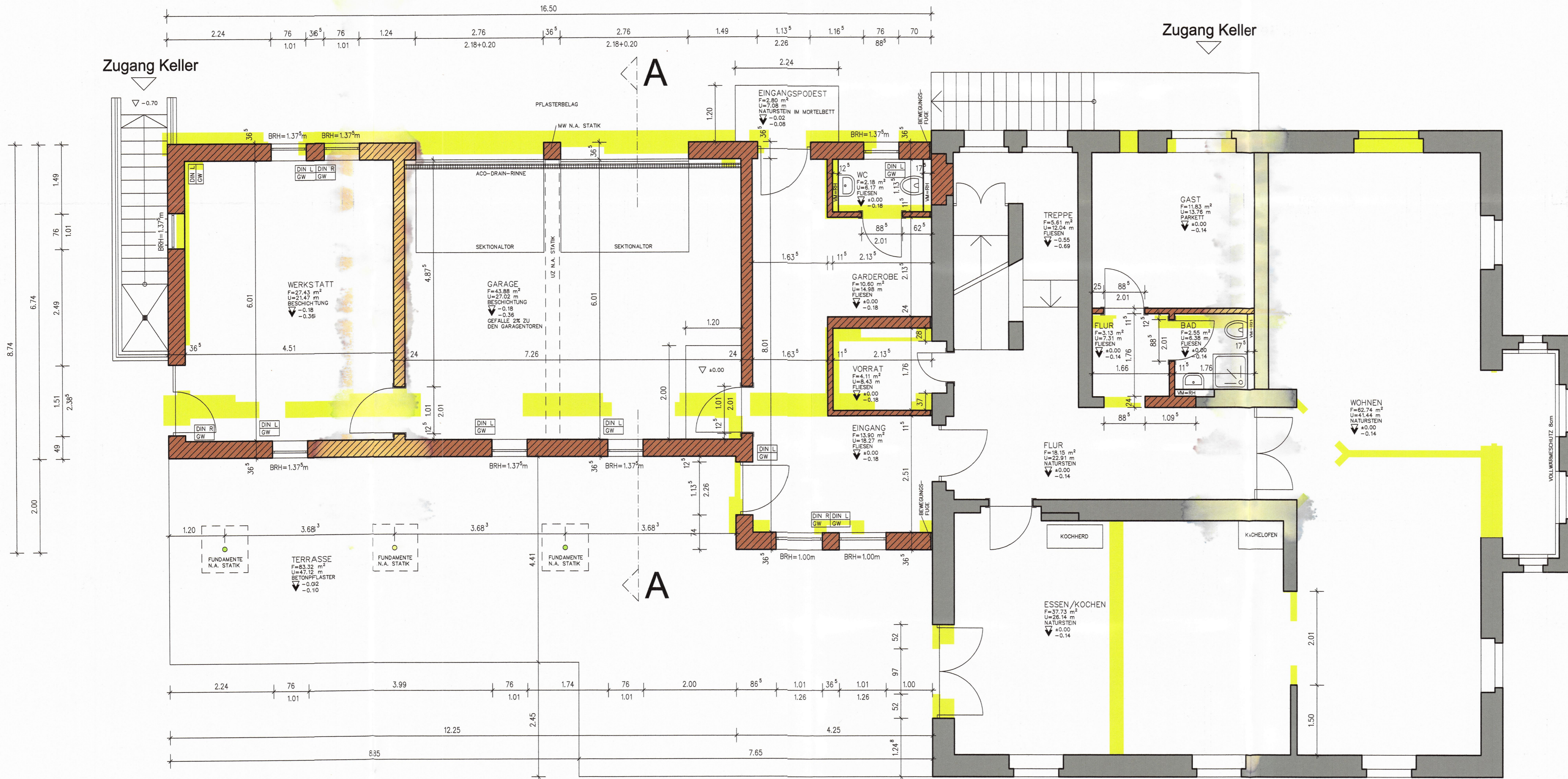
Grundriss EG
